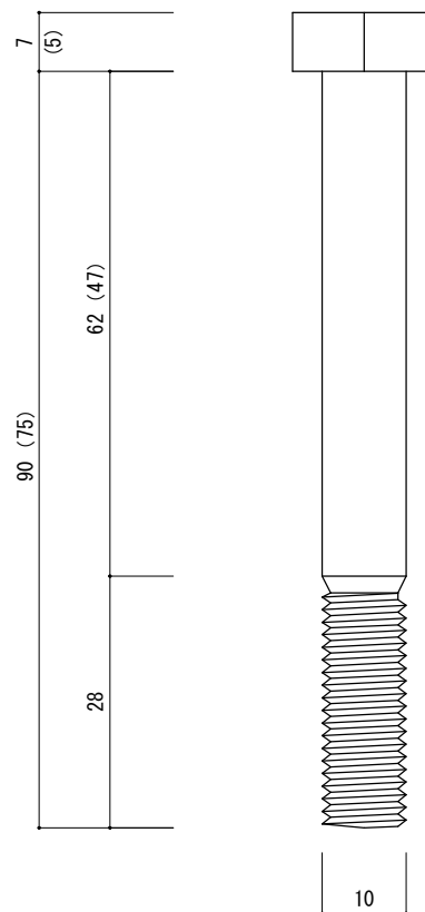
六角ボルトM10 (90 パーキングラバー、カーストップパー用) ※(75)は、エコストップ使用
